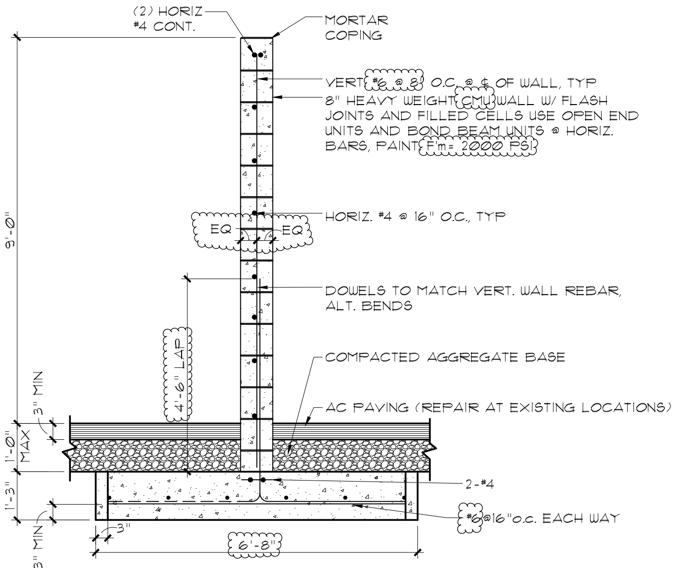
A SECTION SCALE: 1/2" = 1'-0"
