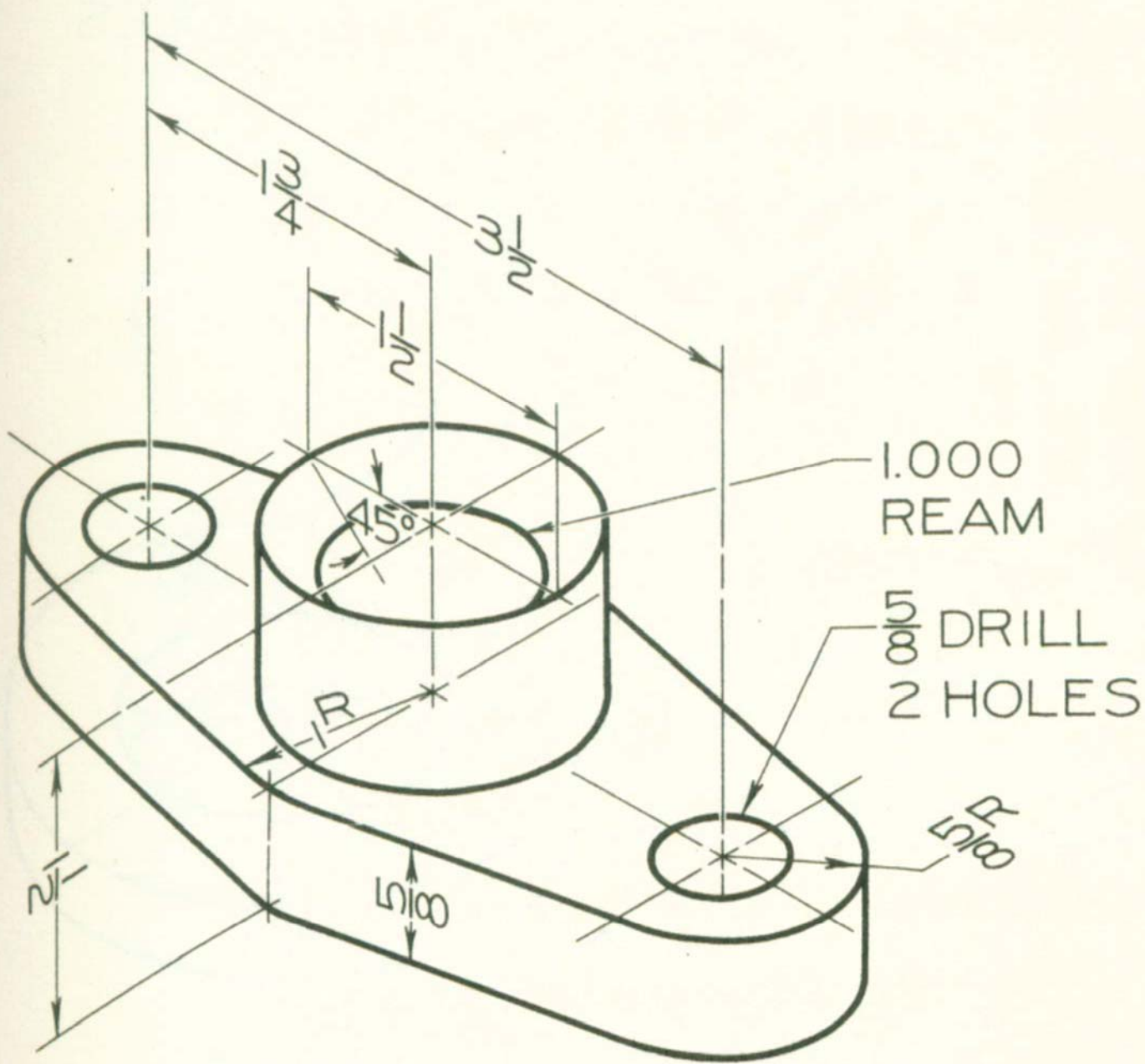
Fig. 259. Packing Gland.*
